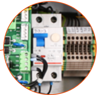
Différentiel de protection pour les tensions supérieures à 48V Leakage protection for voltage >48V
