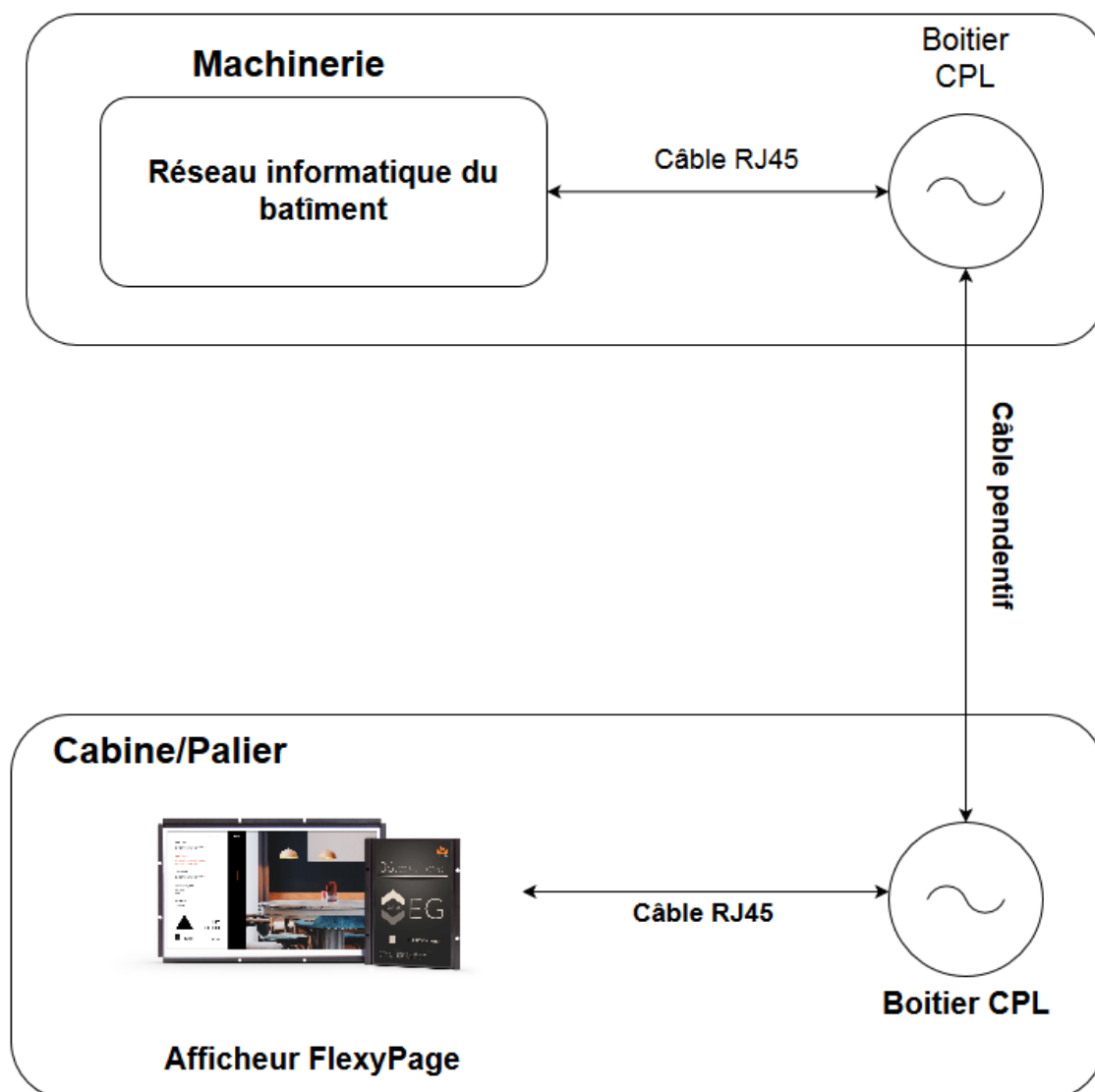
Figure 1 - Installation avec un réseau informatique
